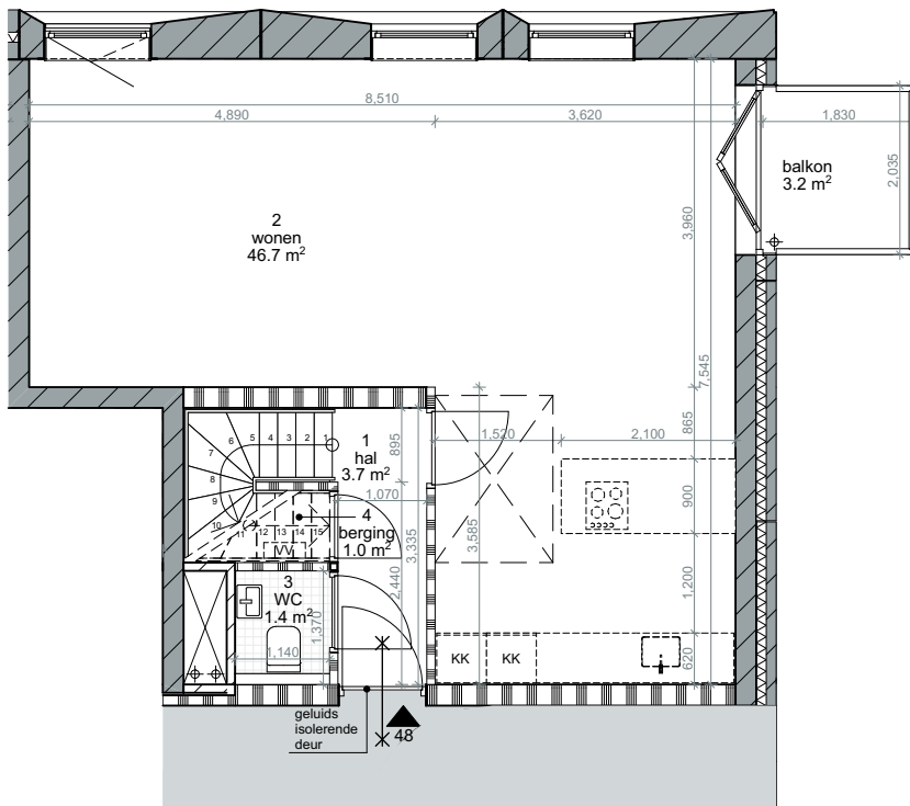
Zesde verdieping
