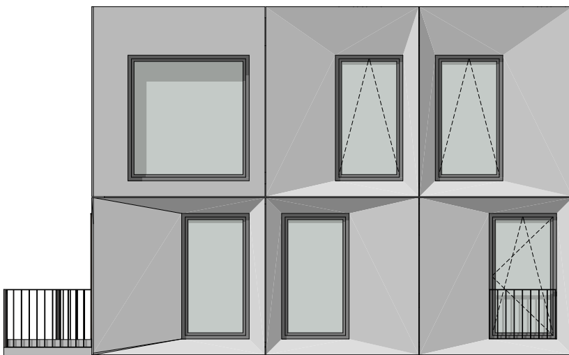
Achtergevel (tuin/parkeren)
