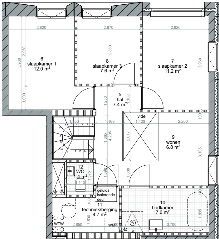
Zevende verdieping
