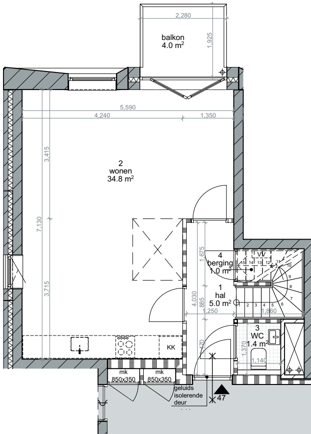
Zesde verdieping
