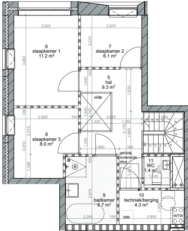
Zevende verdieping
