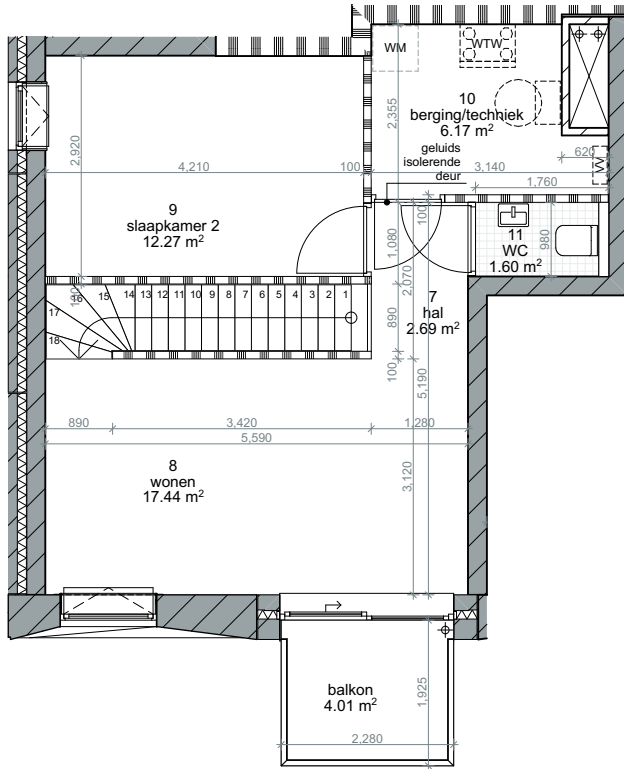
Eerste verdieping
