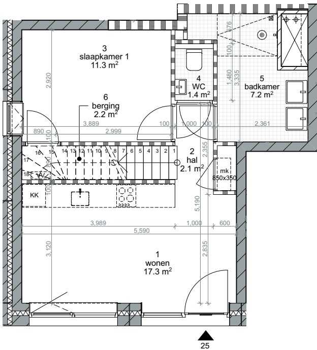
Begane grond
